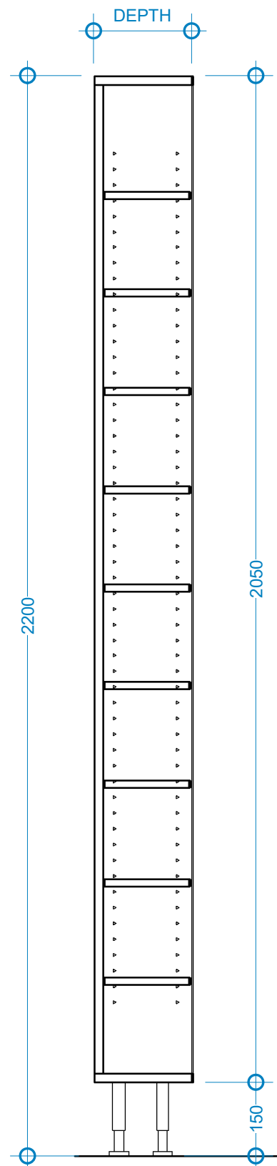
Section 1 1 : 10
