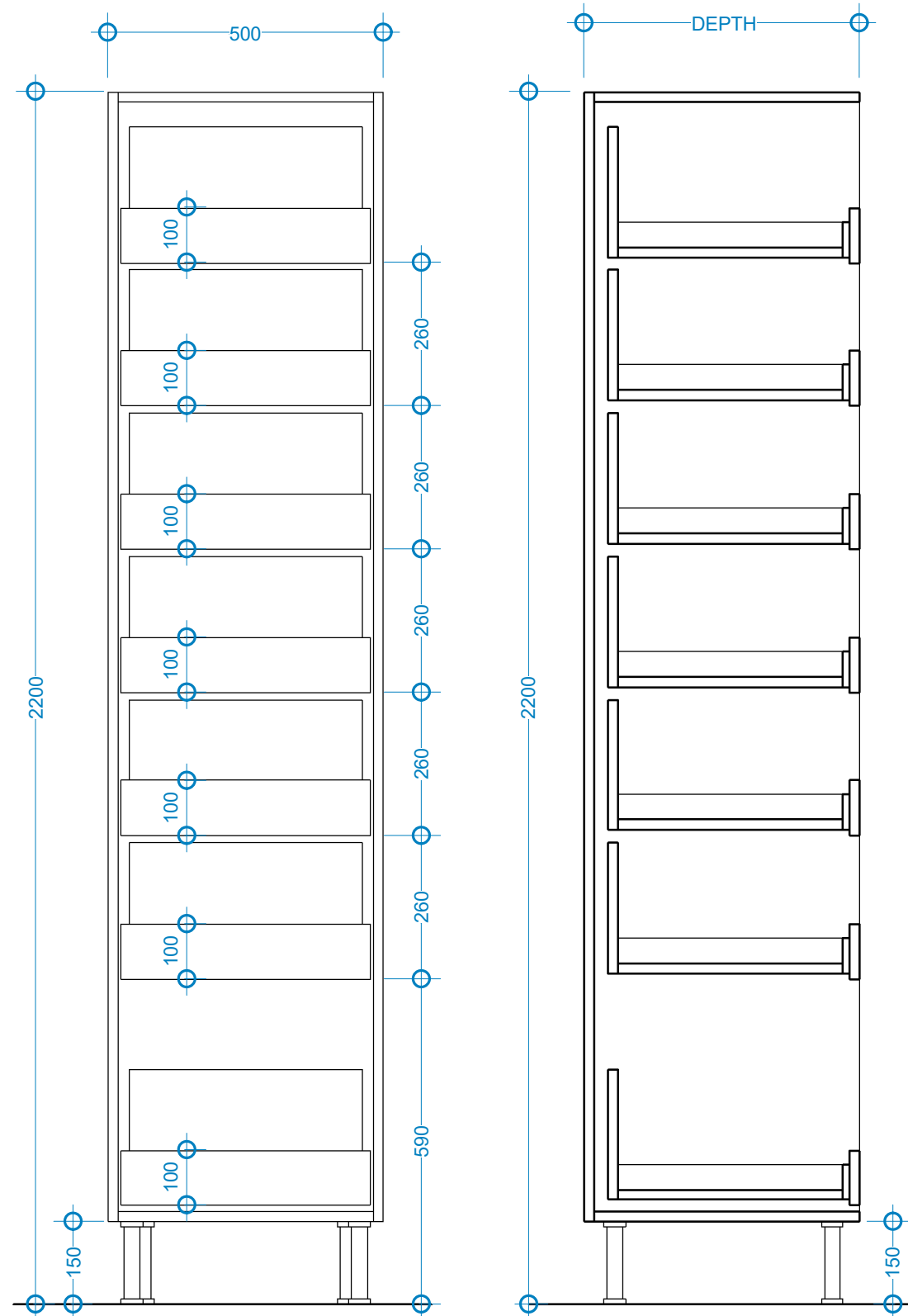
Front 1 : 10
