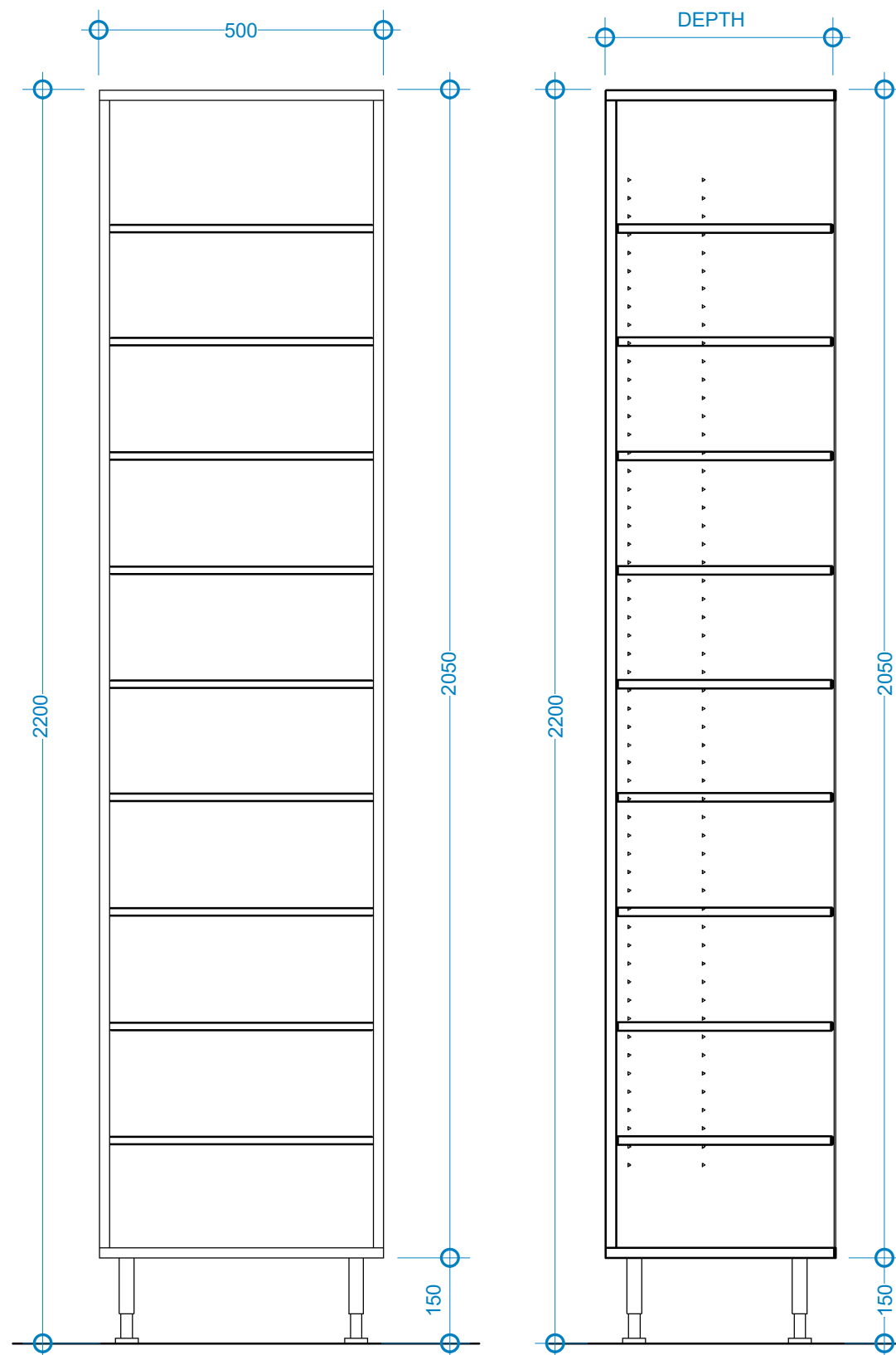
Front 1 : 10
