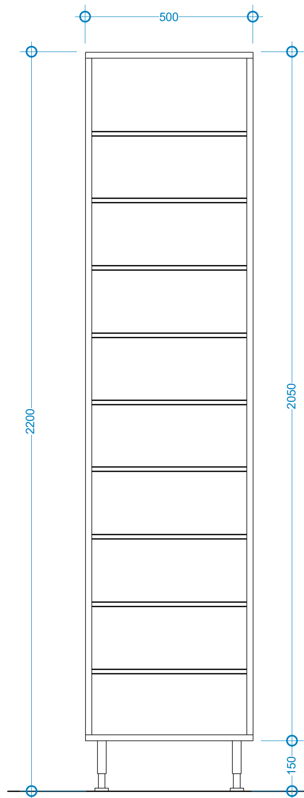
Front 1 : 10
